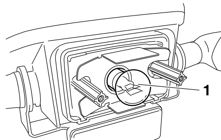
1. Gloeilamp remlicht/achterlicht
