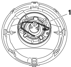
1. Gloeilamphouder
