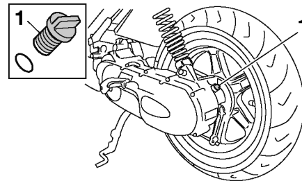
1. Vuldop versnellingsbakolie
