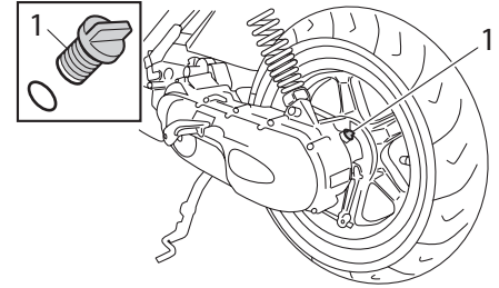
1. Vuldop versnellingsbakolie
