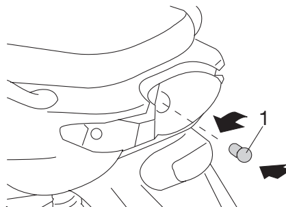
1. Gloeilamp remlicht/achterlicht
