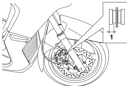
1. Remvoeringdikte
