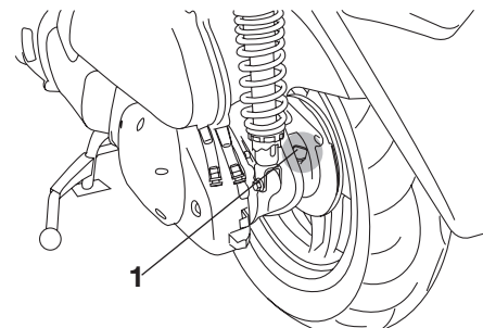
1. Olievulplug eindoverbrenging
