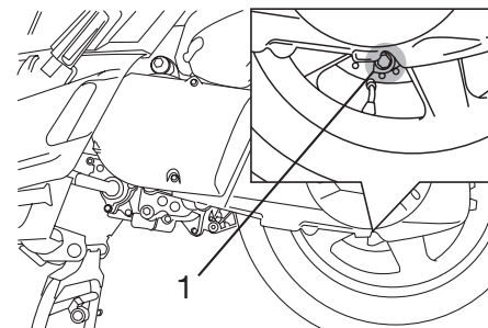
1. Olieaftapplug eindoverbrenging
