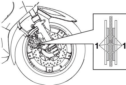
1. Slijtage-indicatorgroef
